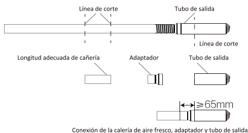
Conexión de la calería de aire fresco, adaptador y tubo de salida
