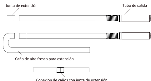
Conexión de caños con junta de extensión
