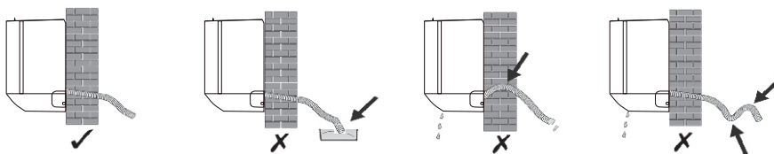
Ubicación de la manguera de drenaje
